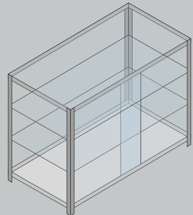
MD.024 / MD.025 Dimensões: 900x950x600 - 900x1250x600mm
