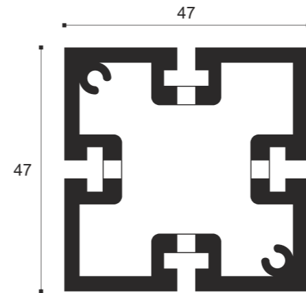
Coluna SU.50 Comprimento: 3000 mm
